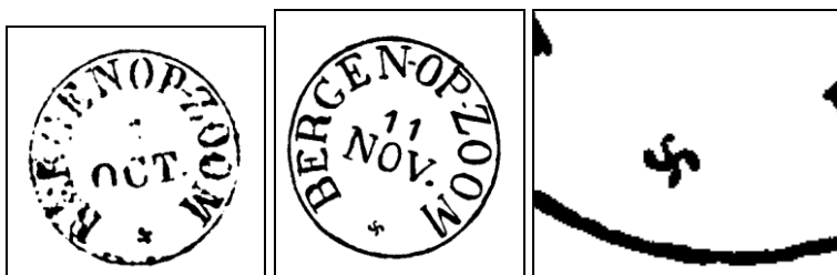
Afbeelding Korteweg
