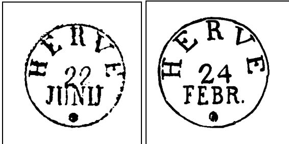
Korteweg
