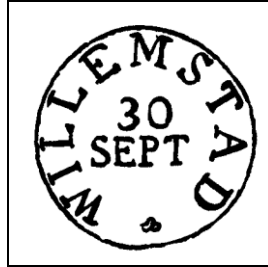
Korteweg
