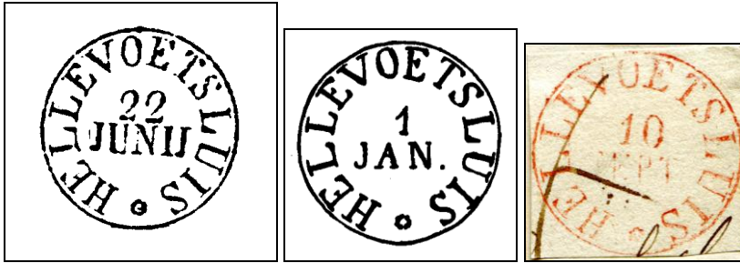
Korteweg
