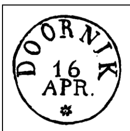
Korteweg
