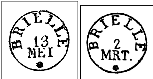
Afbeelding Korteweg
